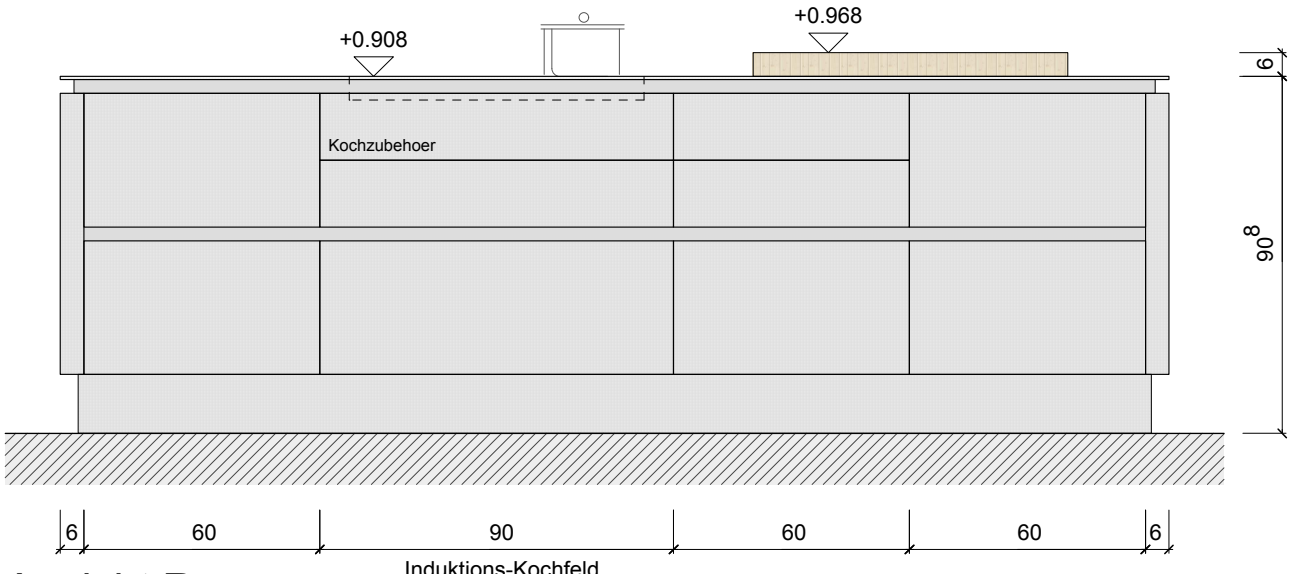
Ansicht B
