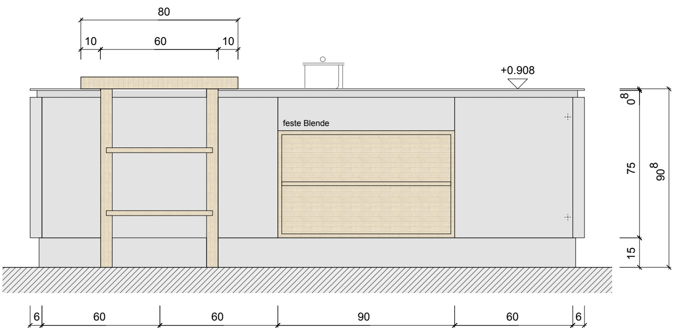
Ansicht C
