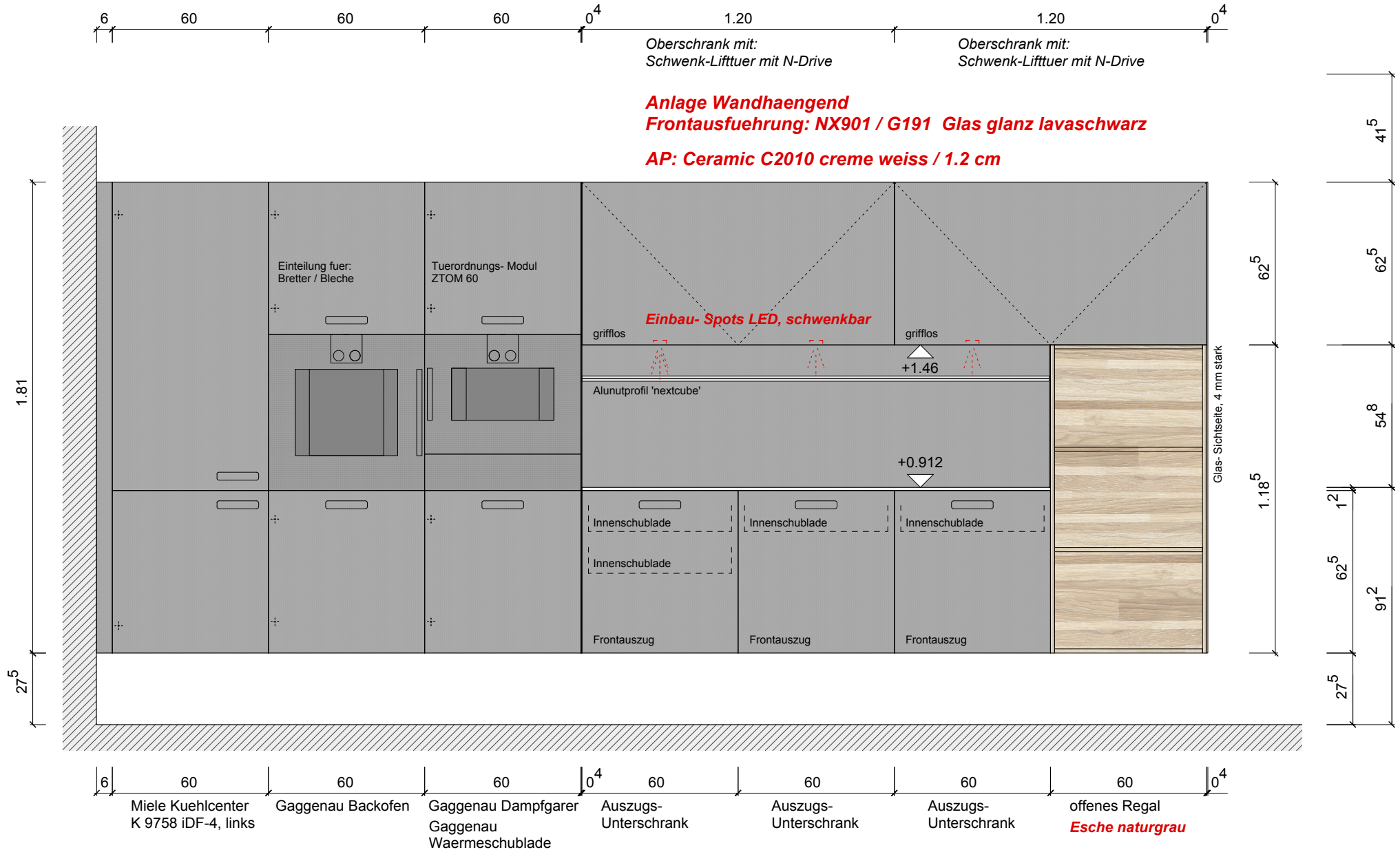
Ansicht A
