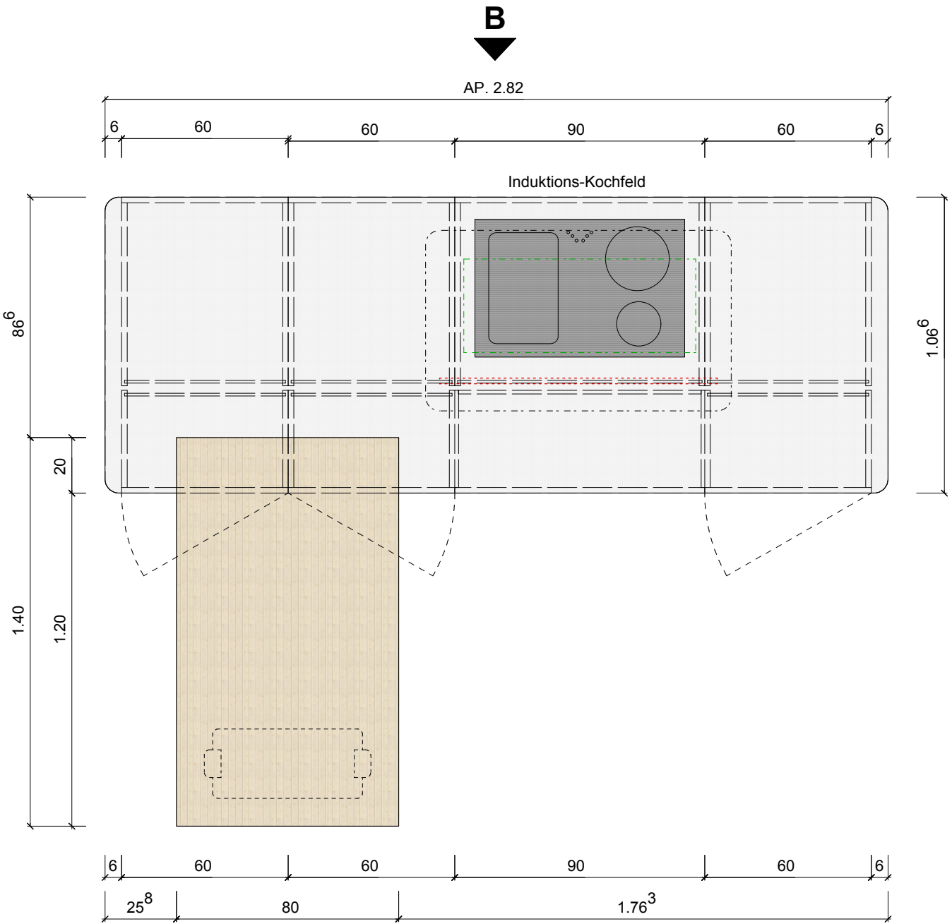
Grundriss AP Insel / Kochen C
