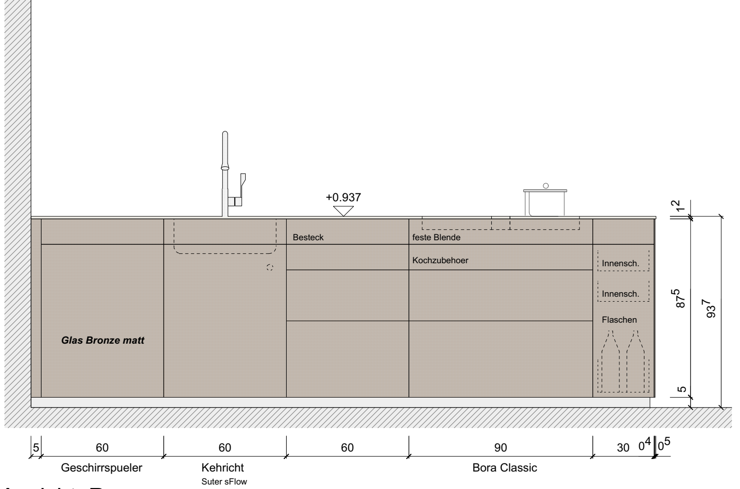
Ansicht B
