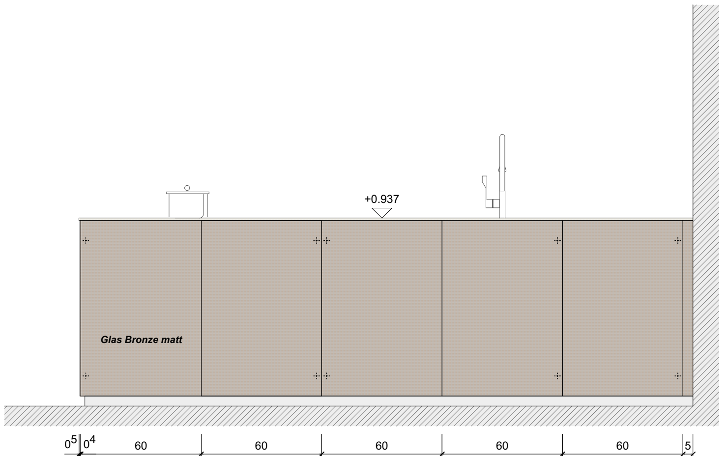
Ansicht C
