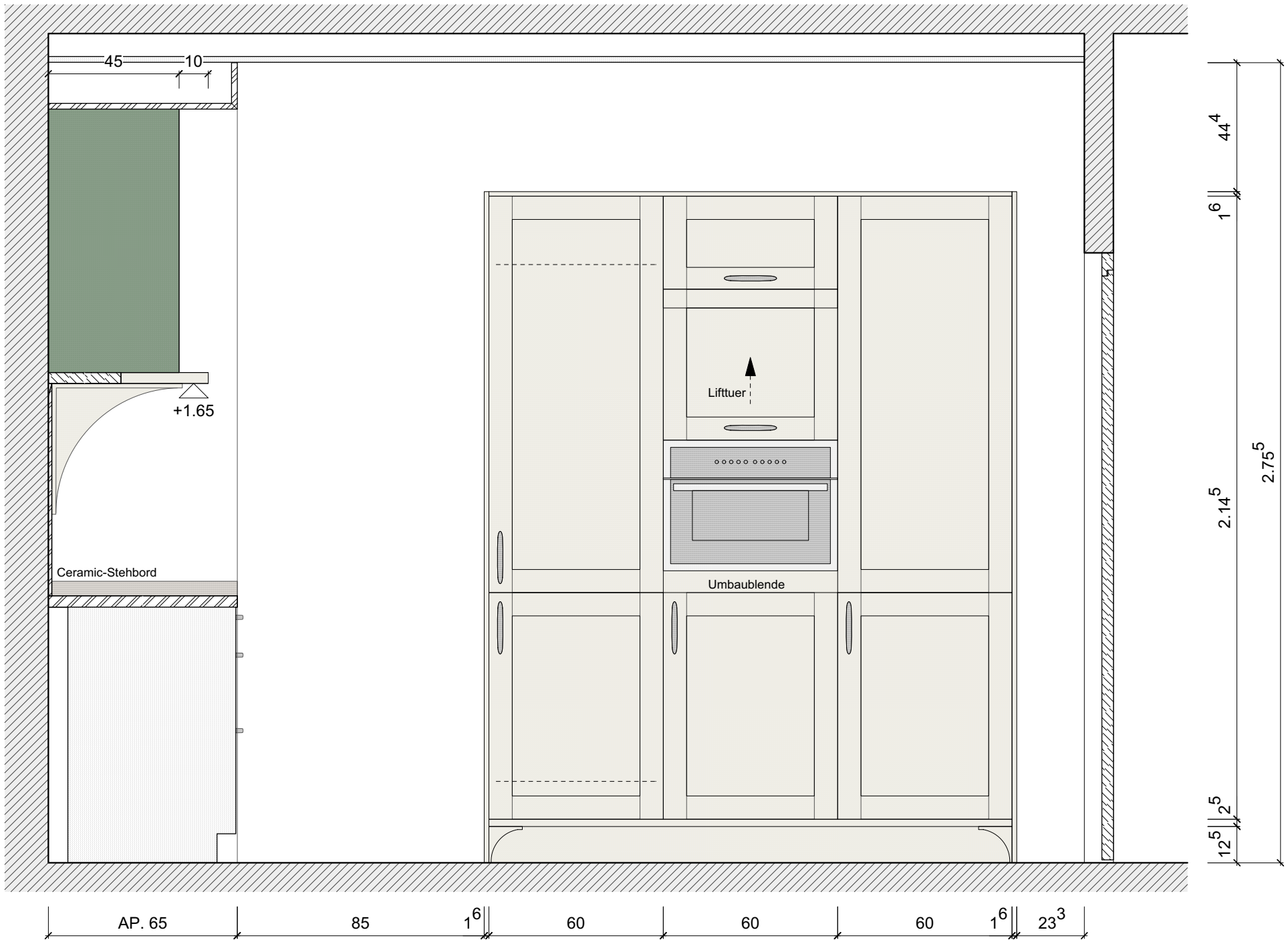
Ansicht B
