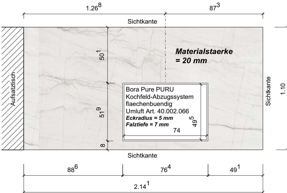
Grundriss AP Insel
