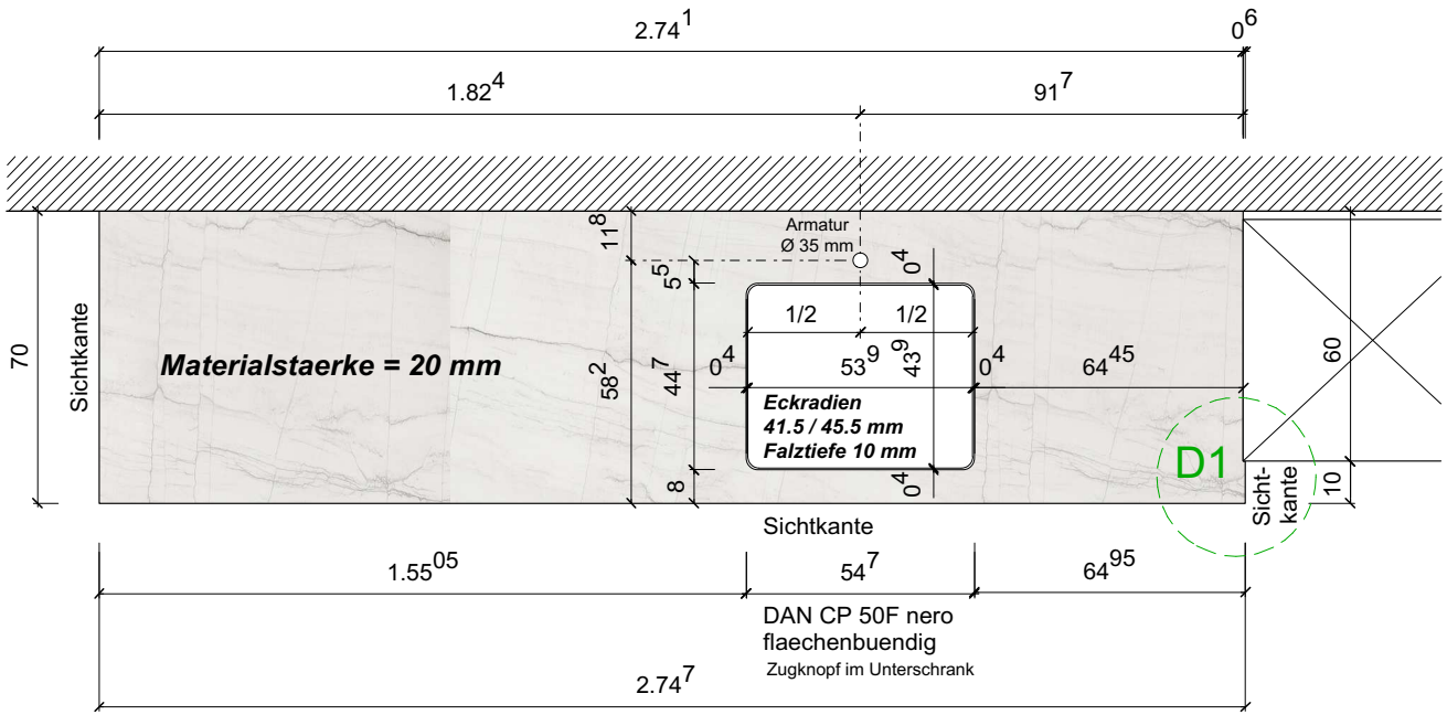
Grundriss AP Spuelen
