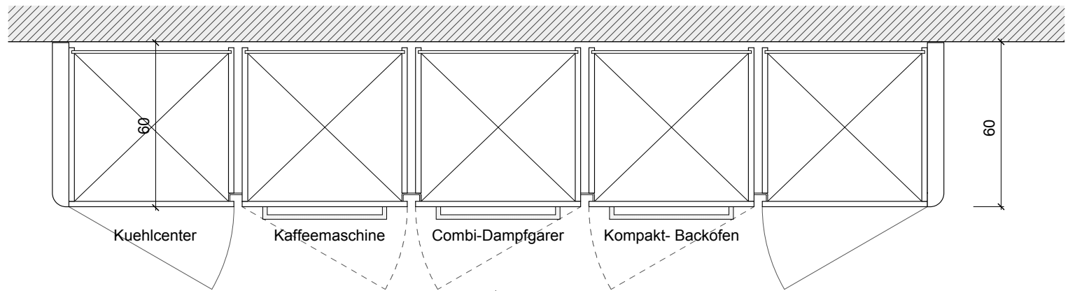
Grundriss Hochschraenke
