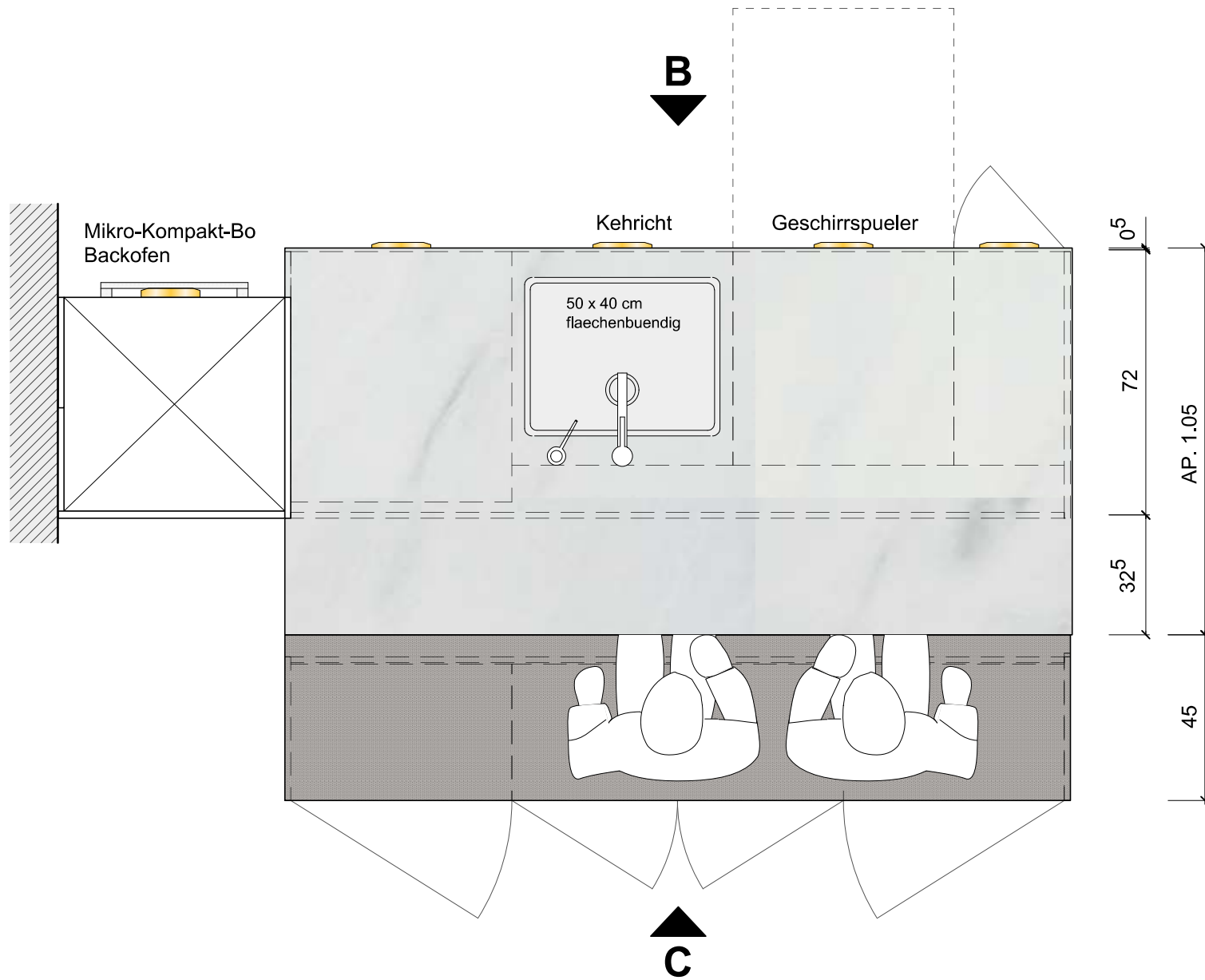
Grundriss Inselanlage / Spülen
