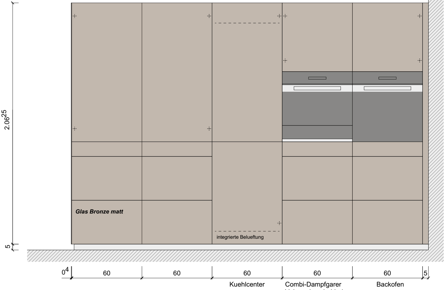
Ansicht A Hochschrankanlage
