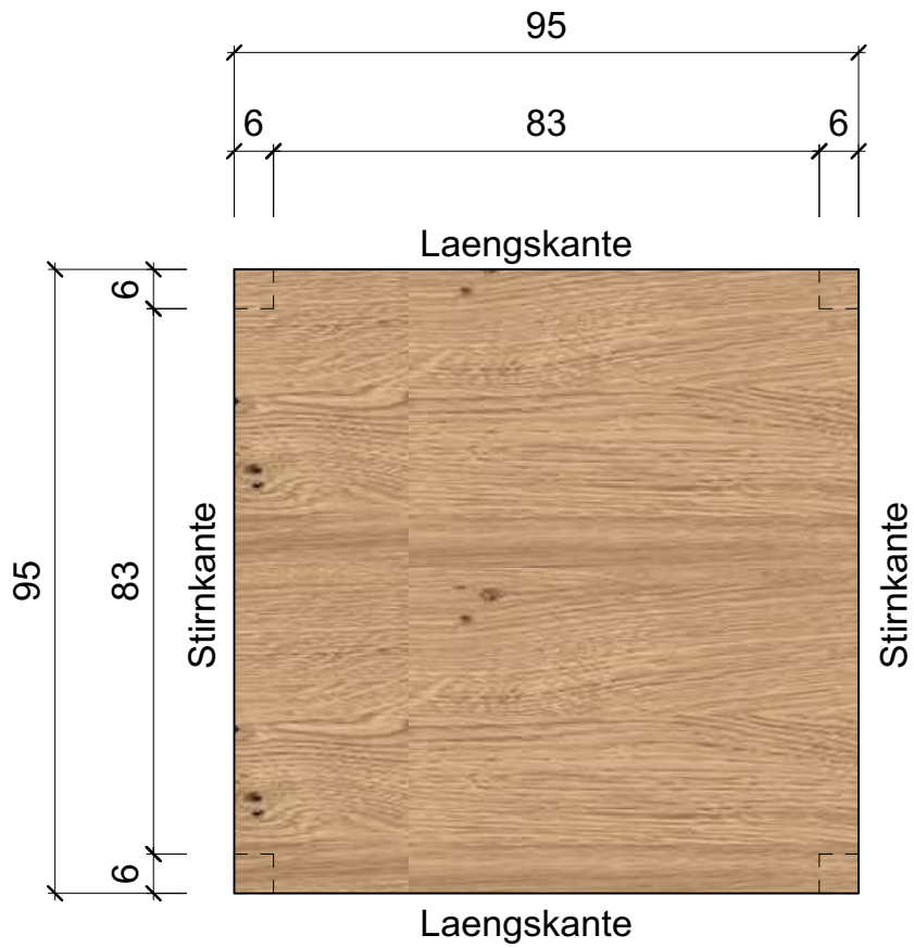
Grundriss Tisch
