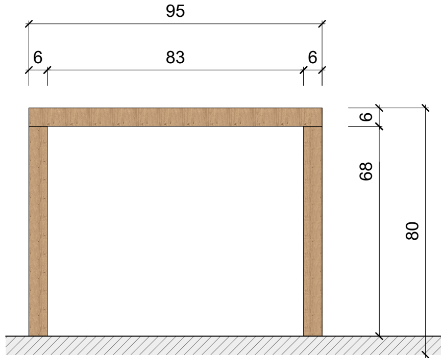
Ansicht Tisch
